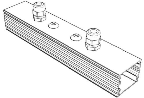
Miteinspeisung aus Aluminium Artikelnr.: 881030
